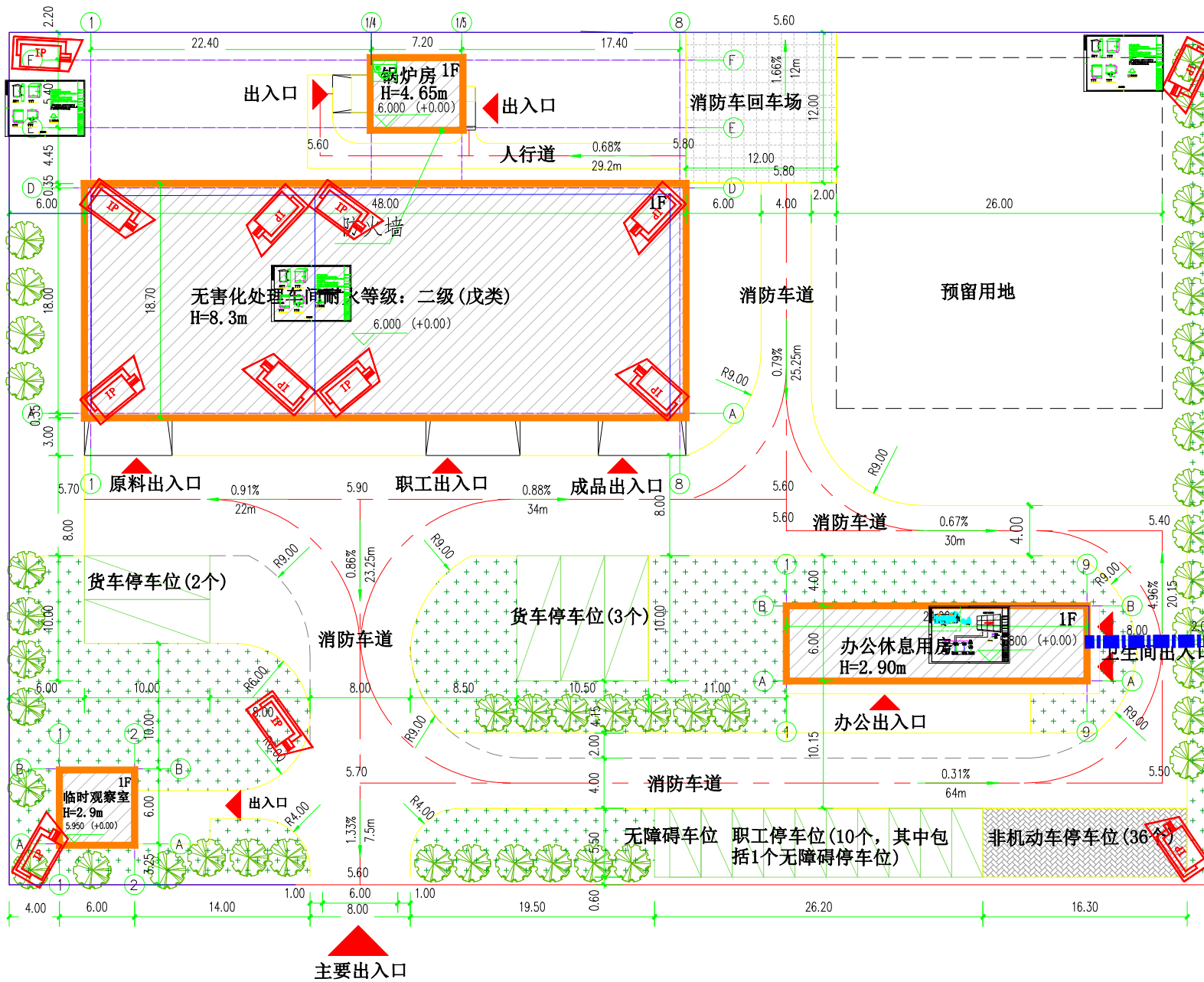
钦州港冷链保税交易中心无害化处理项目安防监控布点图
