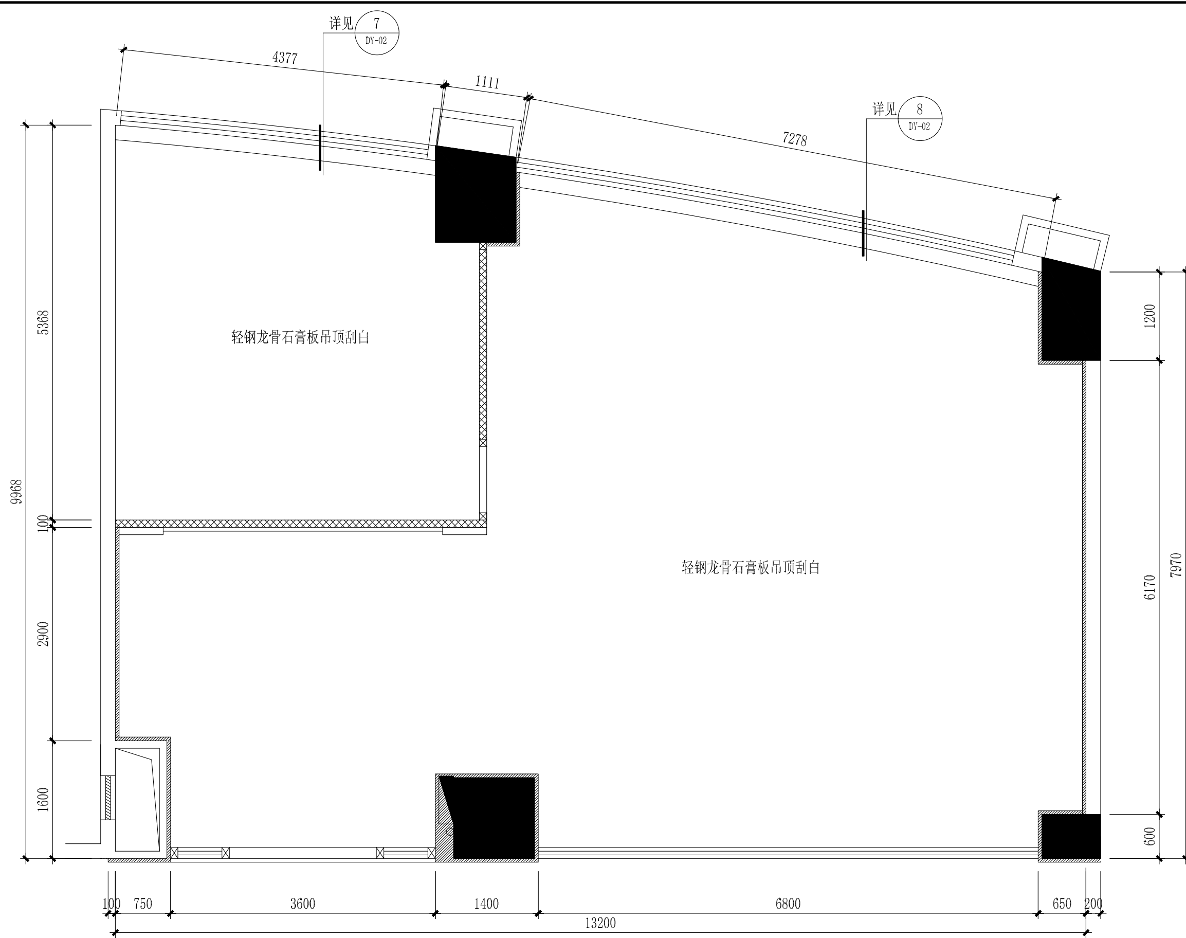
天花吊顶平面图 1:50
