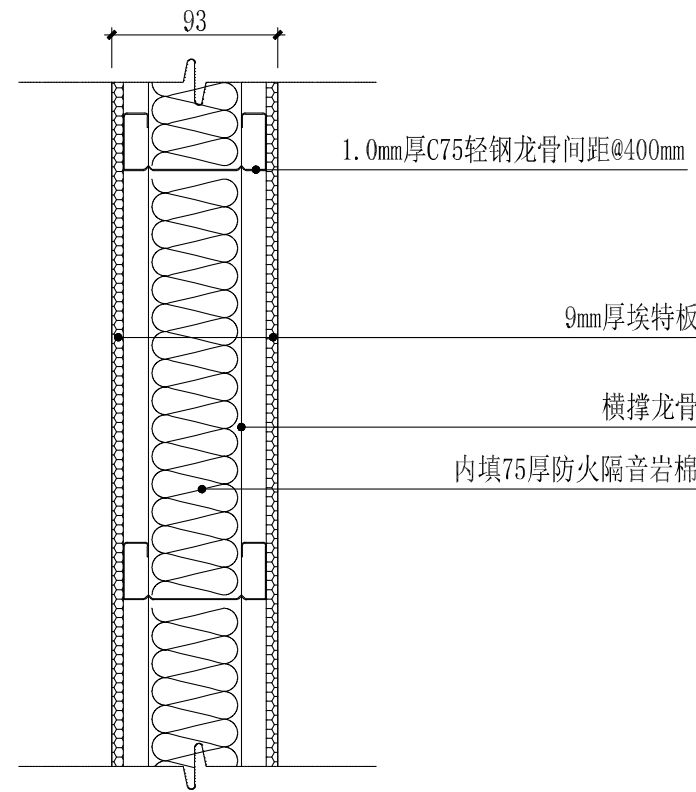
3 大样图 1:5
