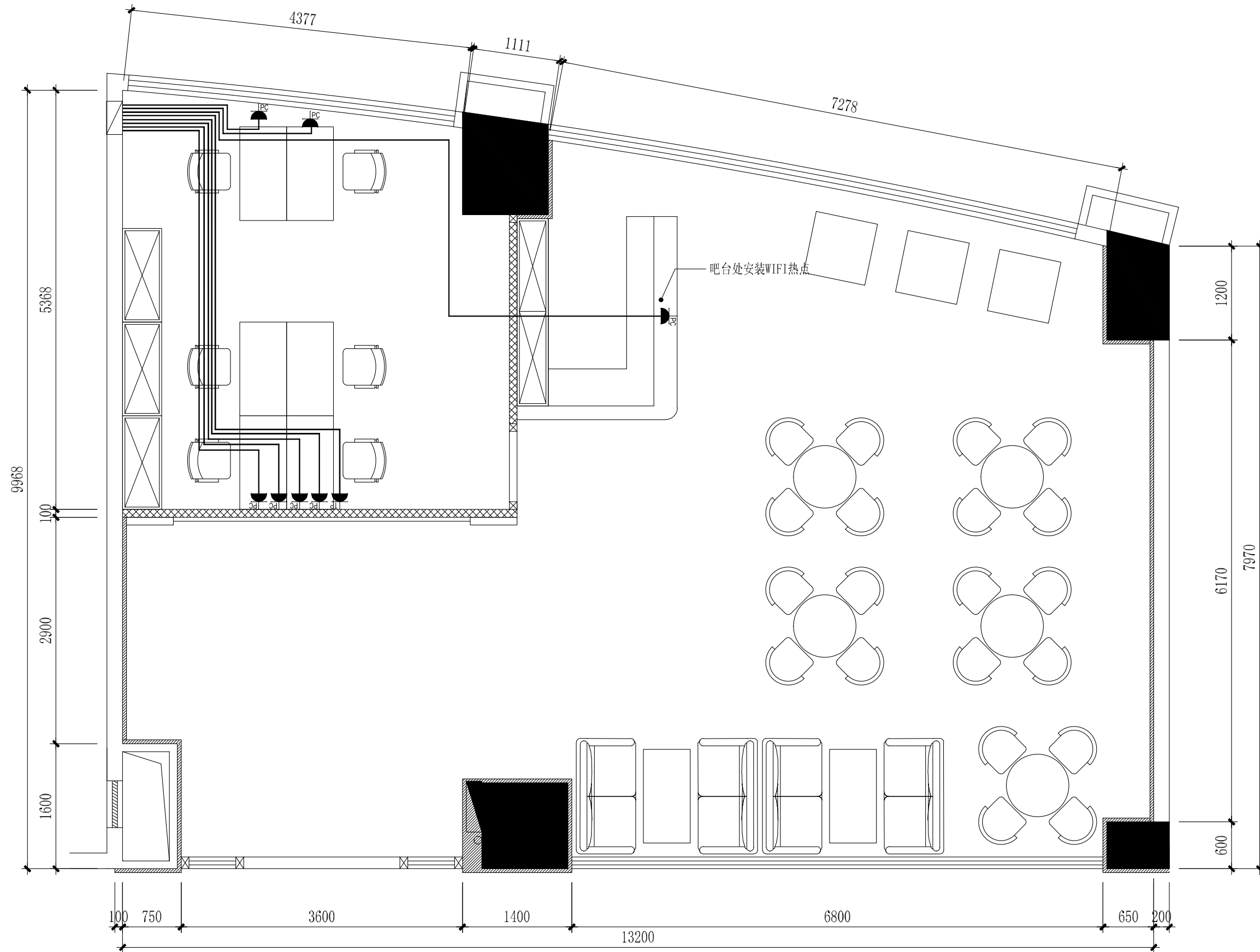
弱电插座布置图 1:50
