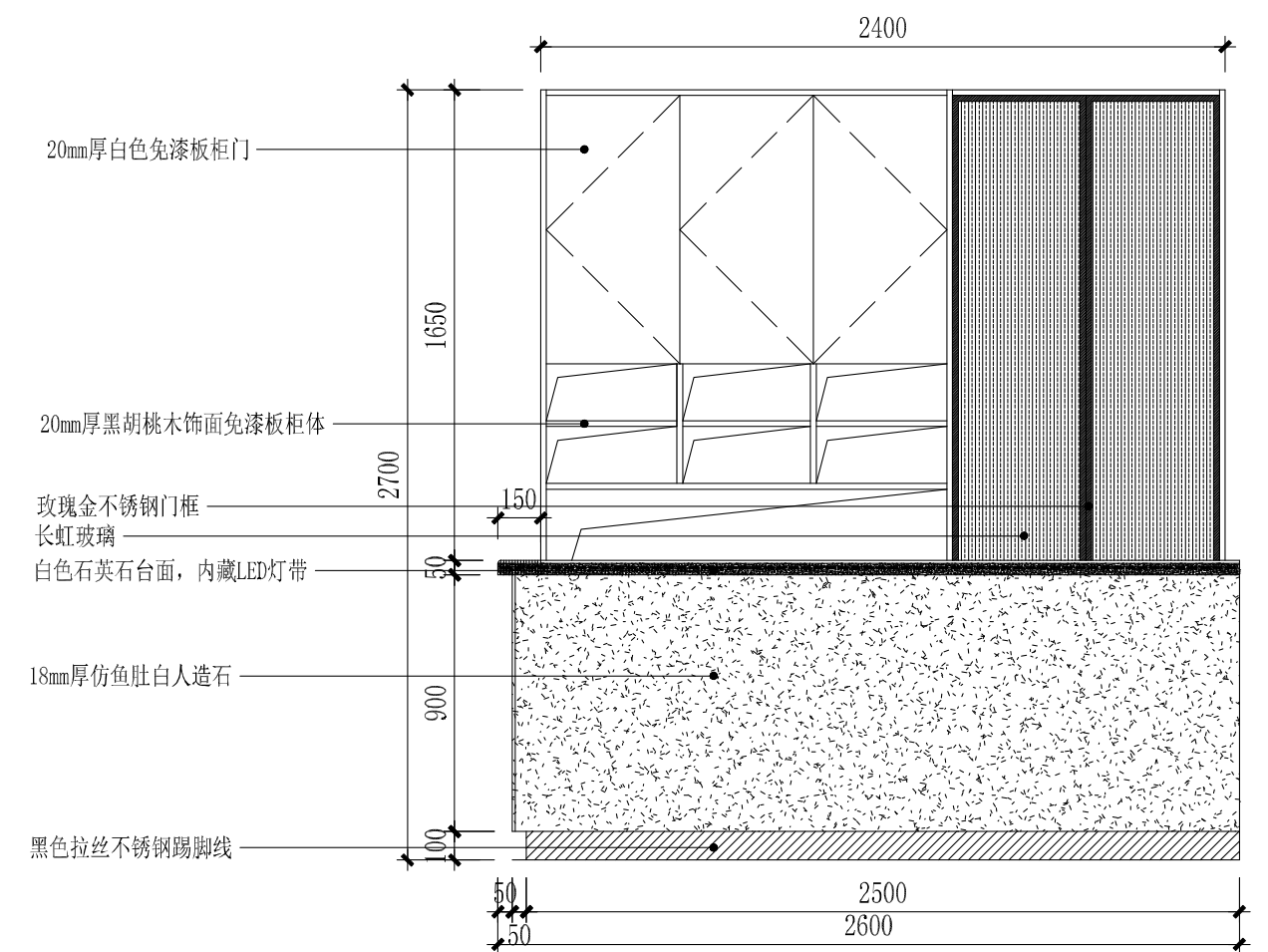
水吧台A立面图 1:25
