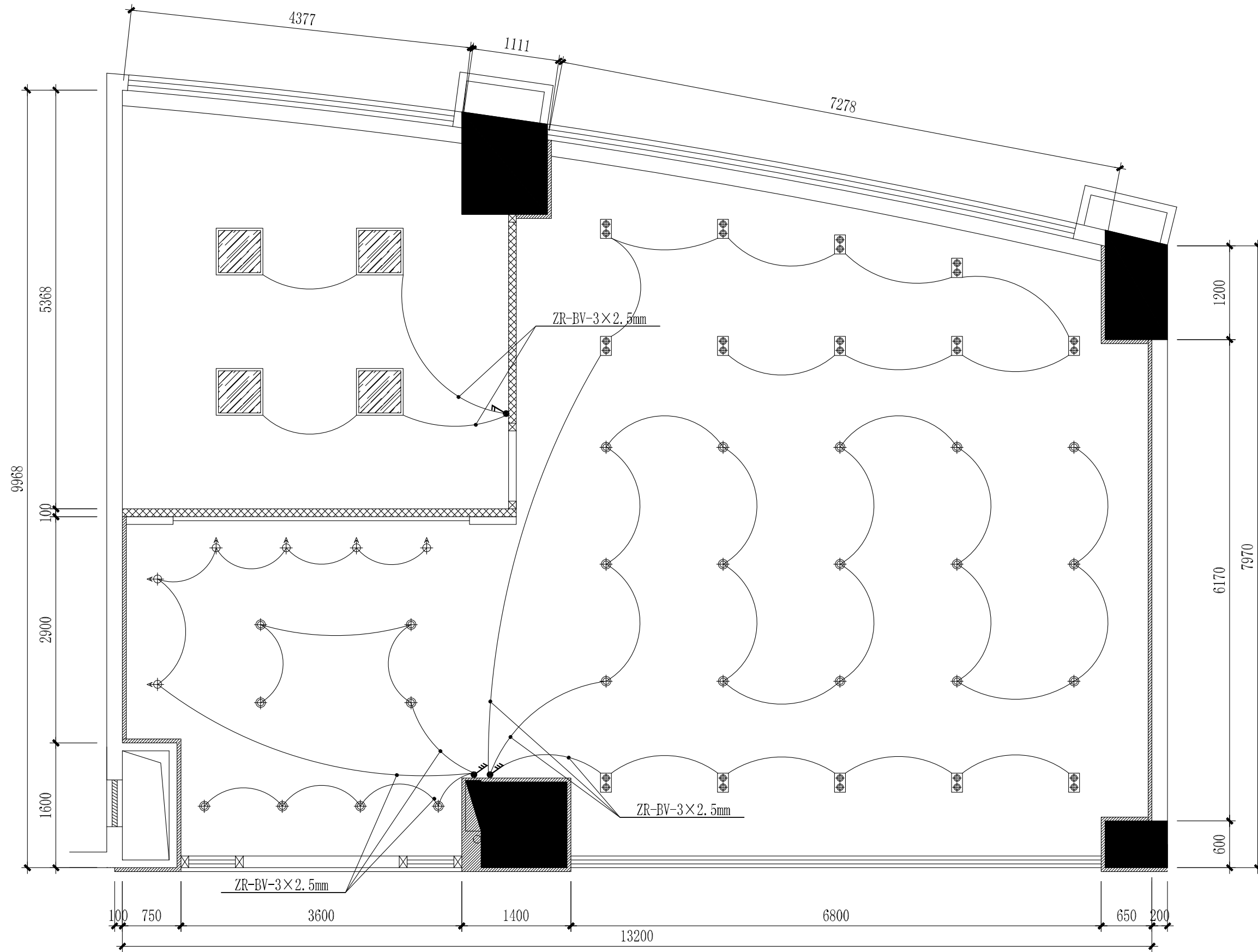
天花灯具连线图 1:50
