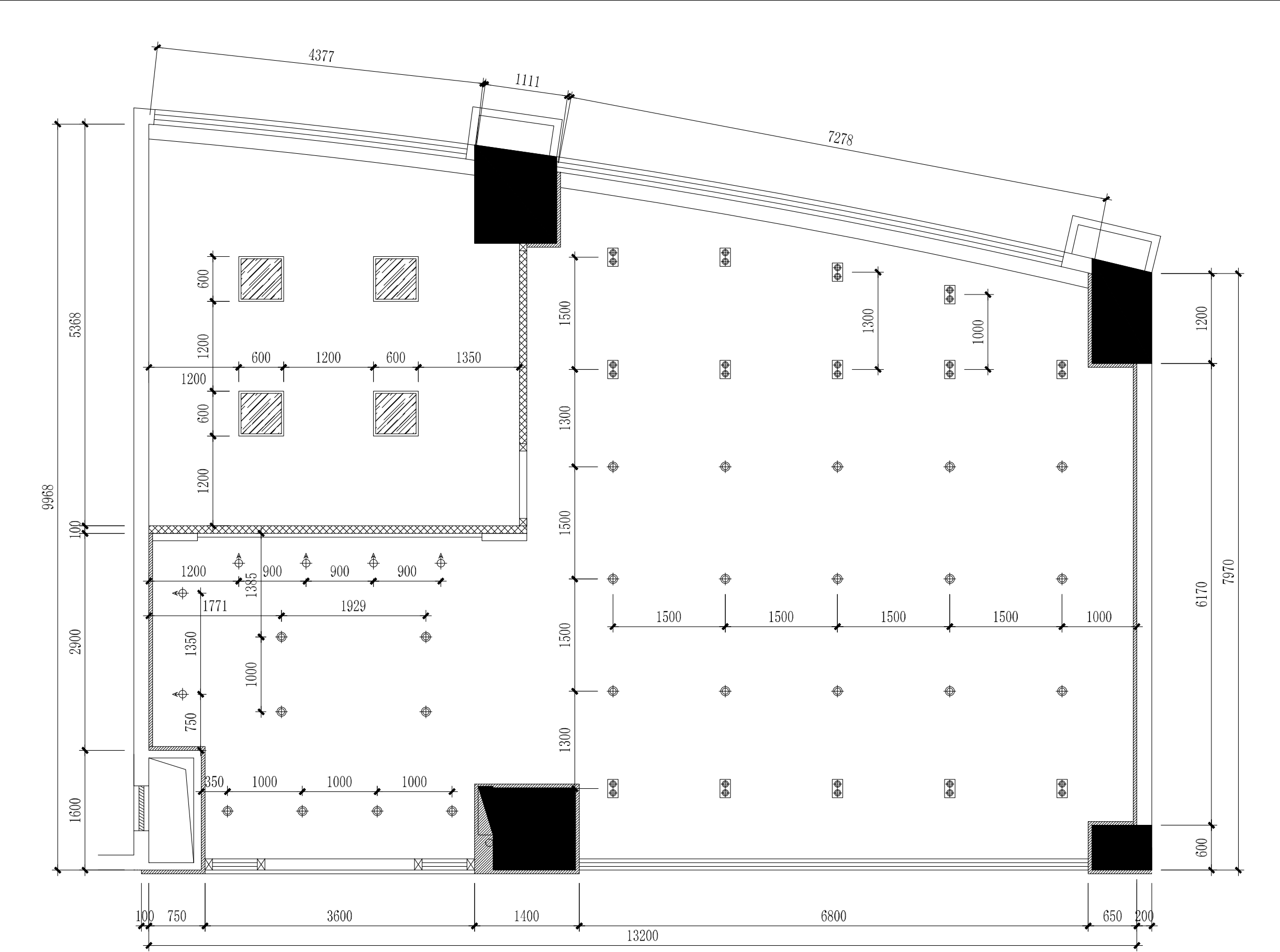
天花灯具布置图 1:50
