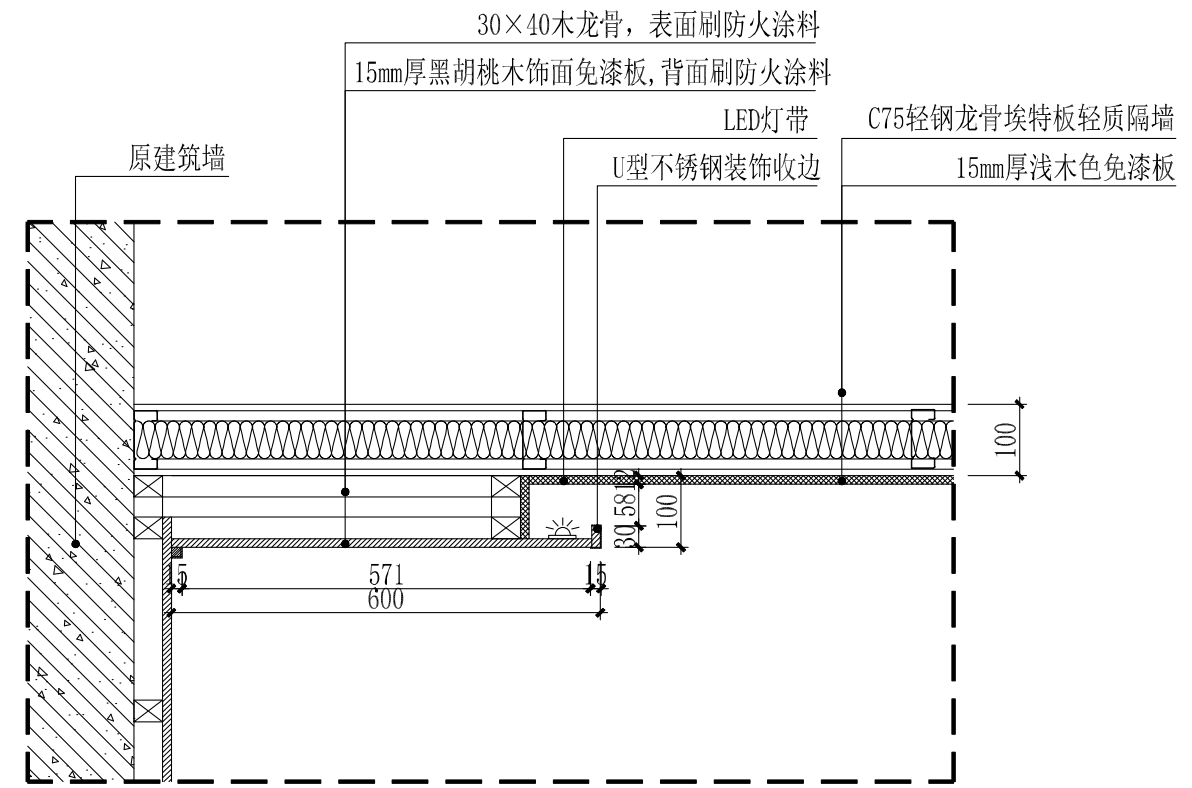
10 大样图 1:10
