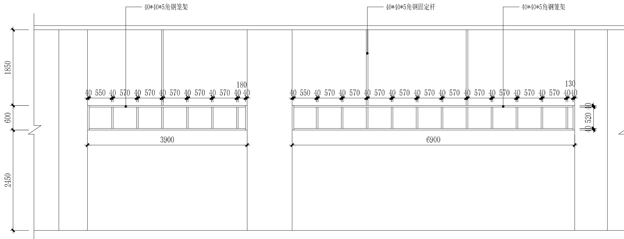
大门门头钢架结构图 1:50
