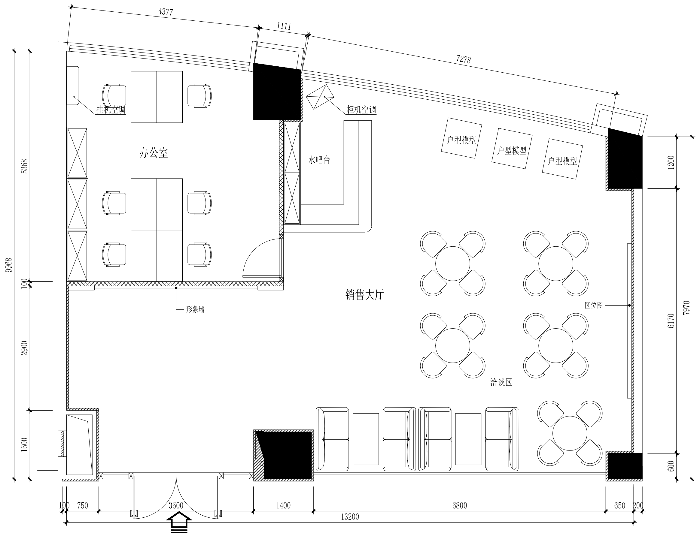
平面布置图 1:50
