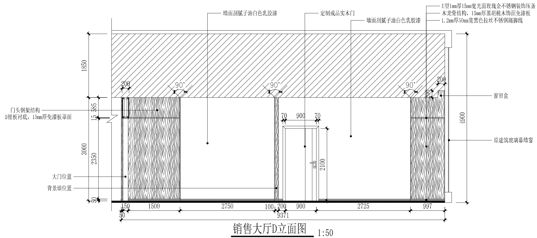
销售大厅C立面图 1:50
