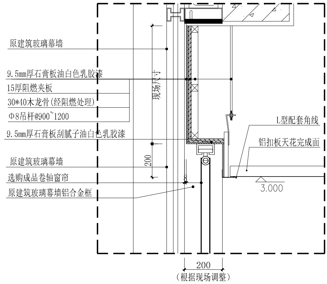
7 大样图 1:10
