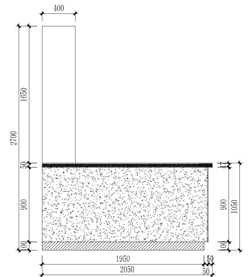
水吧台B立面图 1:25
