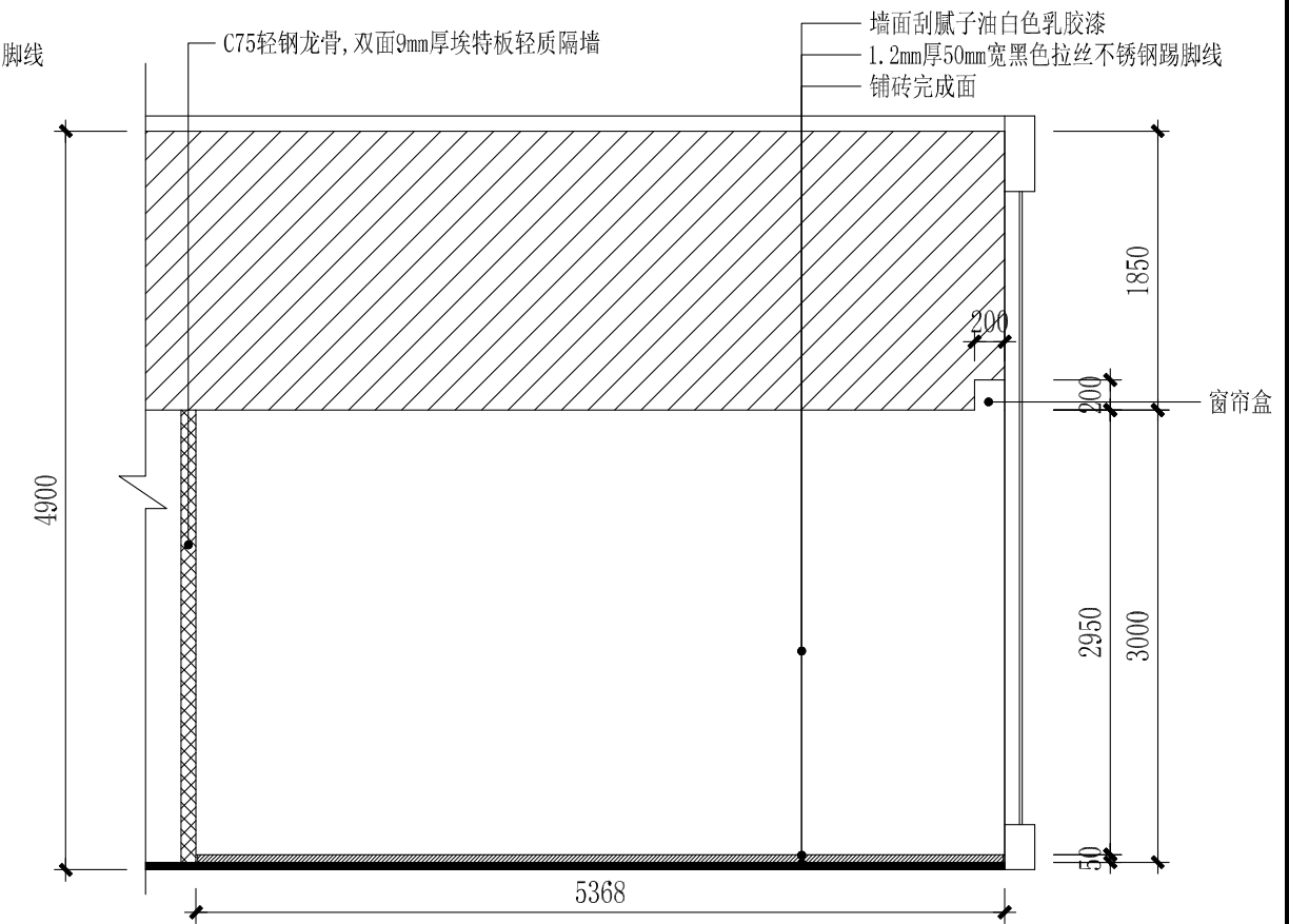
办公室D立面图 1:50
