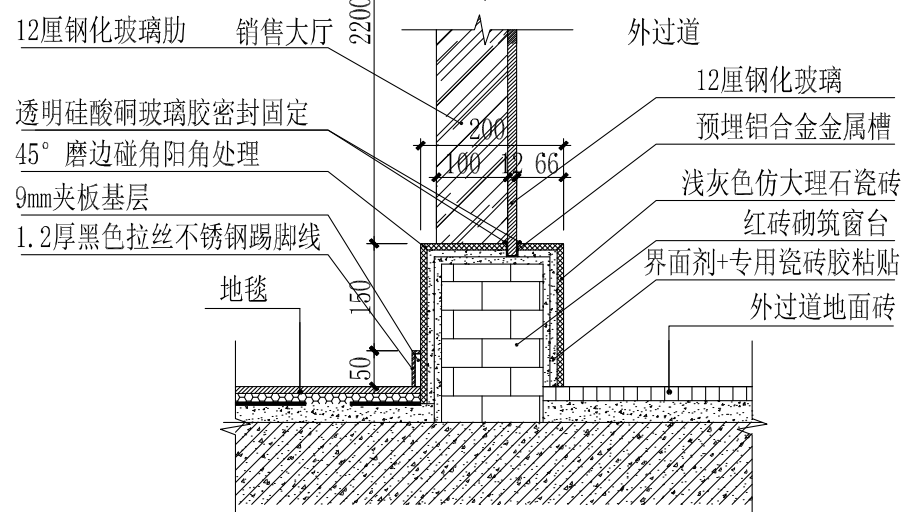
1 大样图 1:10
