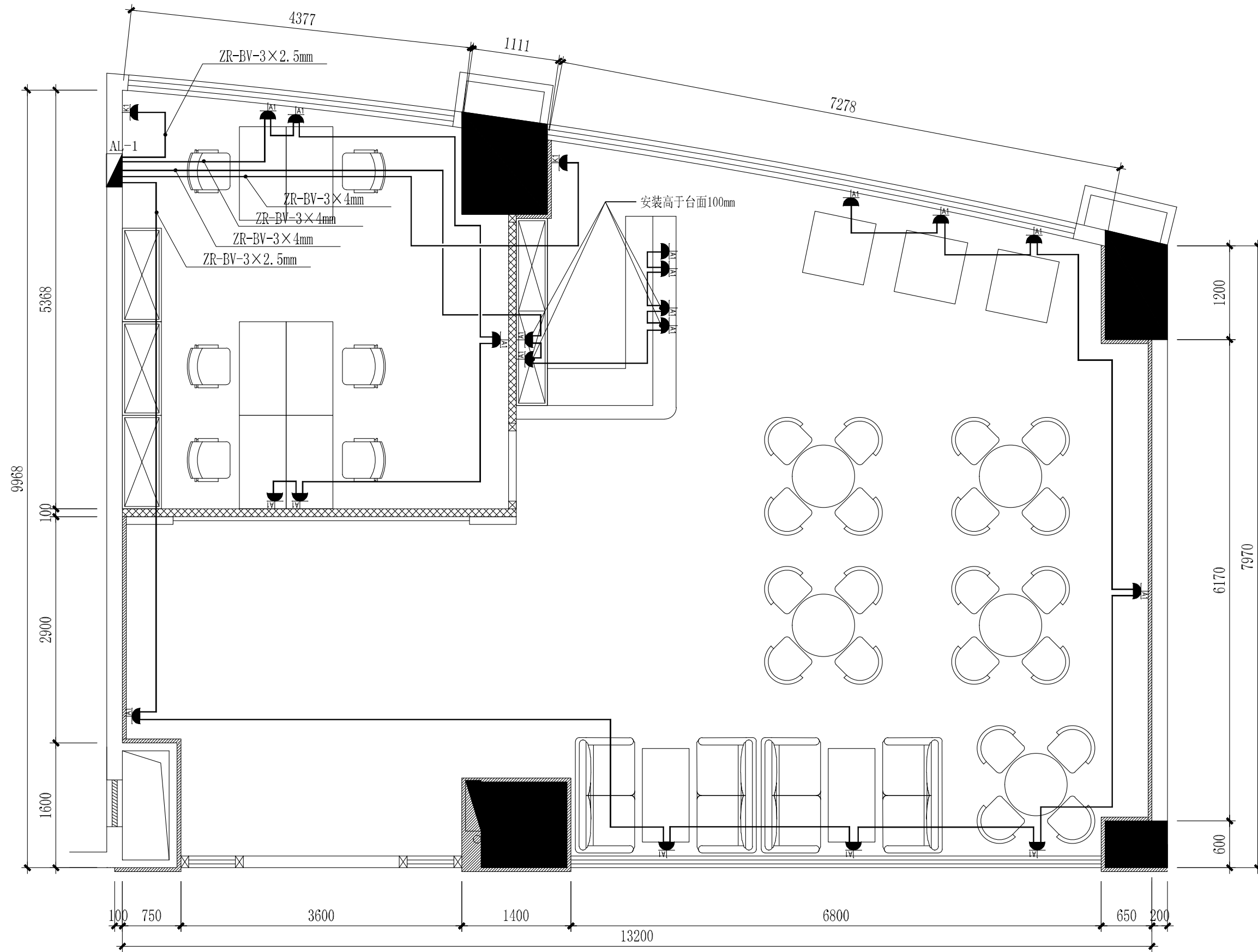
强电插座布置图 1:50
