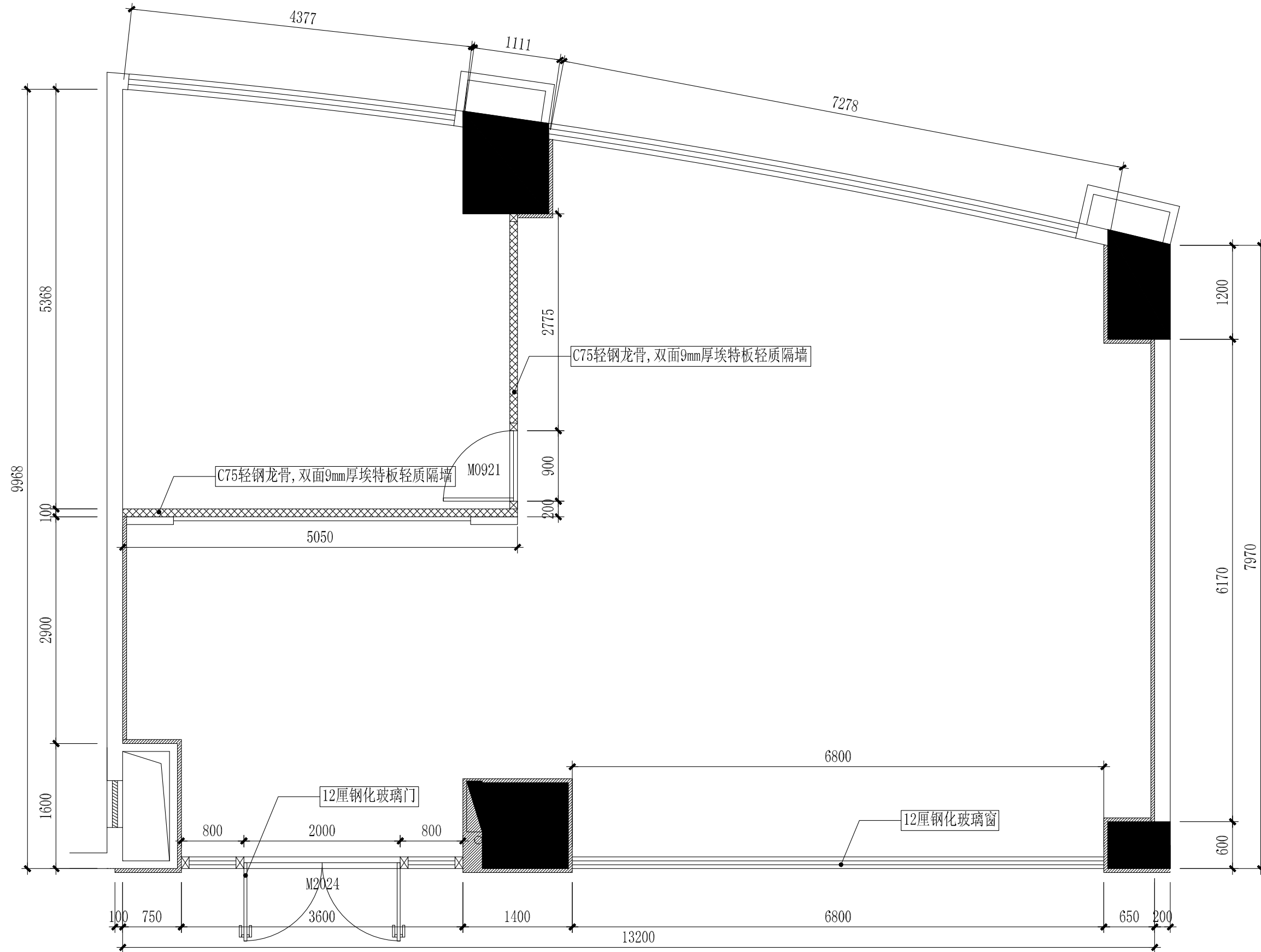
新建隔墙平面图 1:50
