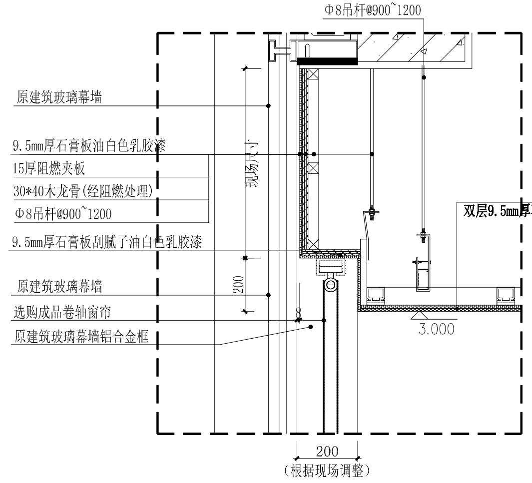
8 大样图 1:10
