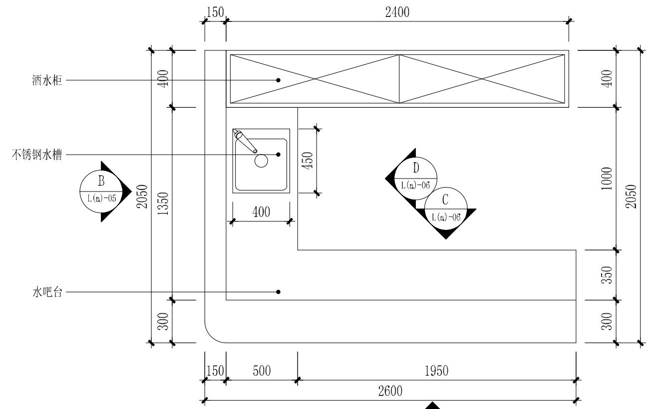
水吧台平面图 1:25
