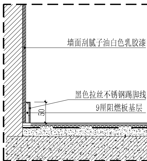
5 大样图 1:10
