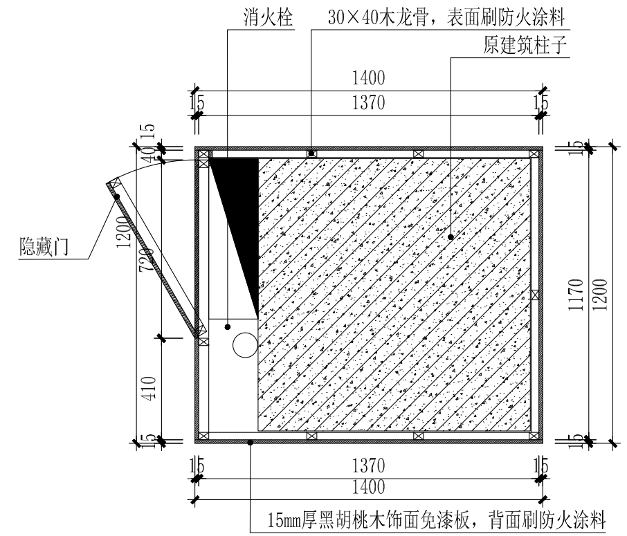
9 大样图 1:20
