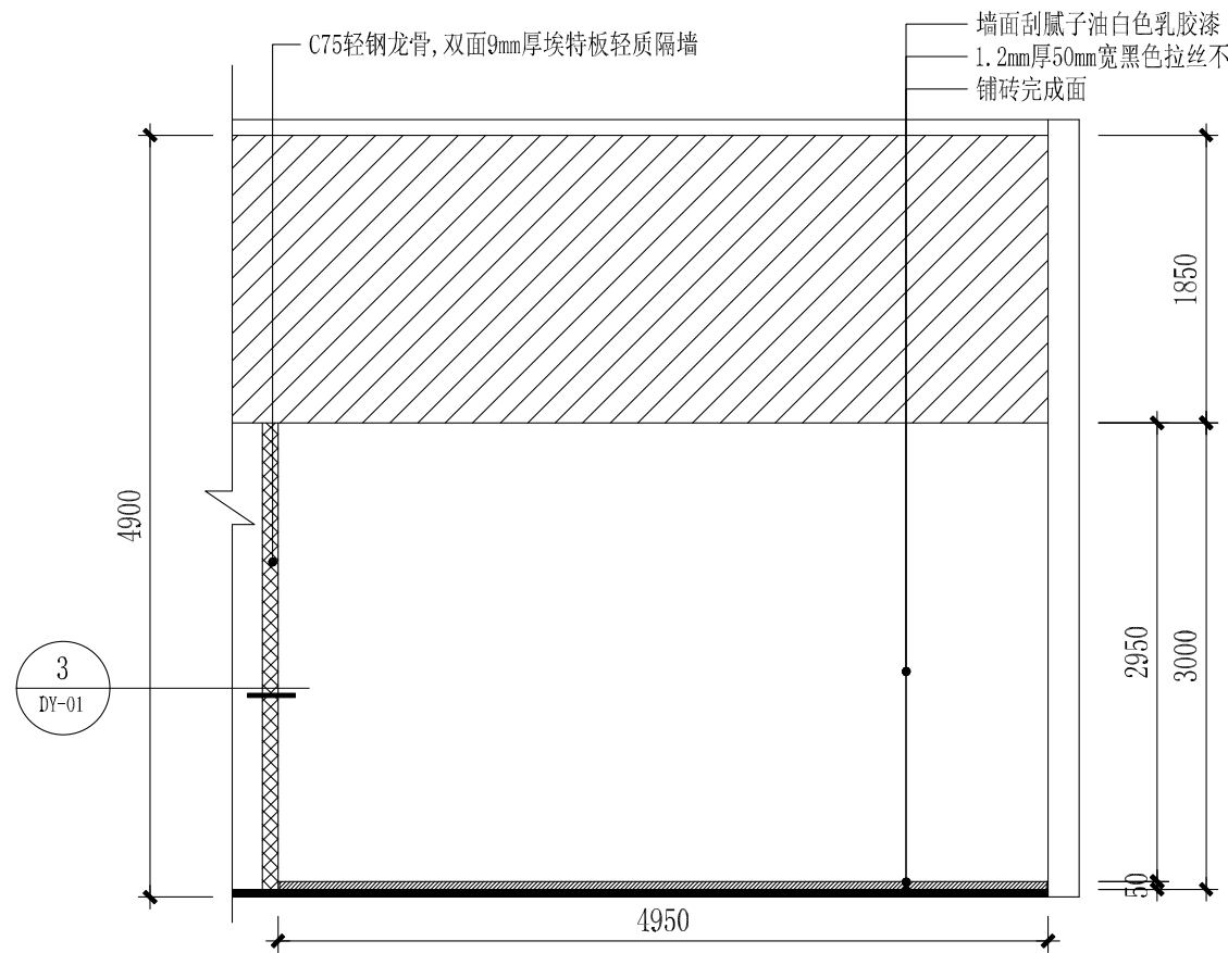
办公室C立面图 1:50
